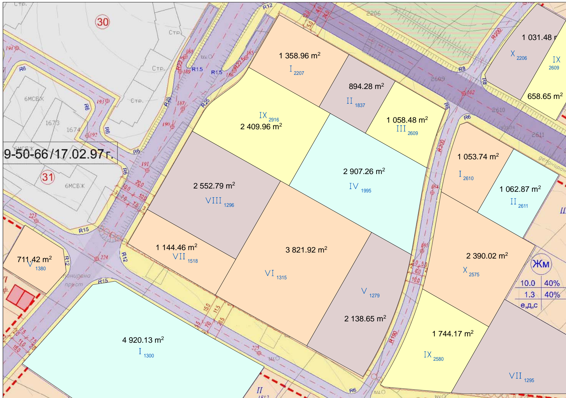
Схема на прилагане на чл. 16, ал. 1÷5 ЗУТ
