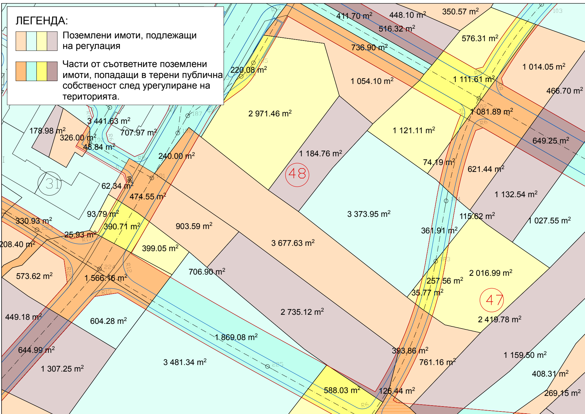
Схема на поземлени имоти по кадастрална карта при прилагане на чл. 16, ал. 1÷5 ЗУТ По материали от НАГ - София и ГИС - София ЕООД
